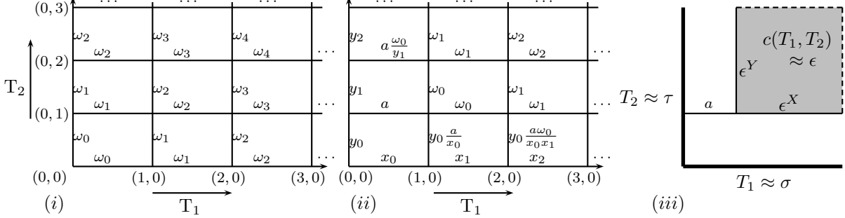
Figure 1. Weight diagrams of \Theta(W_\omega) and W_{(\alpha,\beta)} with c(W_{(\alpha,\beta)}) \cong \Theta(W_\omega) ; and Berger measure diagram of W_{(\alpha,\beta)} with c(W_{(\alpha,\beta)}) \cong \Theta(W_\omega) , respectively. (Schéma des poids de \Theta(W_\omega) et W_{(\alpha,\beta)} avec c(W_{(\alpha,\beta)}) \cong \Theta(W_\omega) ; et schéma de la mesure de Berger de W_{(\alpha,\beta)} avec c(W_{(\alpha,\beta)}) \cong \Theta(W_\omega) , respectivement.)
